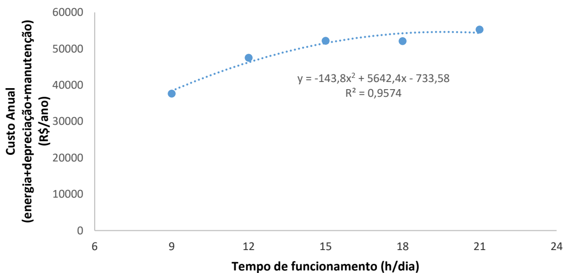
Figura 5. Valores do custo anual (energia + depreciação + manutenção) do sistema de irrigação em função do seu tempo de funcionamento diário.
