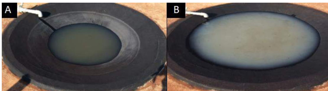
Figura 3. Reator solar de tronco cônico invertido operando com lâminas de 0,10 (A) e 0,20 (B) metros de profundidade (ALVES, 2015).
