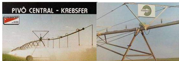
Figura 11. Catálogo pivôs Krebs e Irrigabrás.
