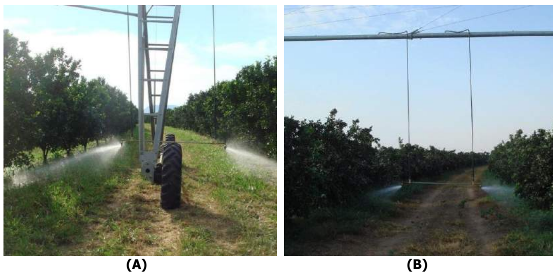
Figura 8. Pivô central. Aspersor tipo Spray direcional irrigando citros: instalados junto à torre (A) e ao vão (B).
