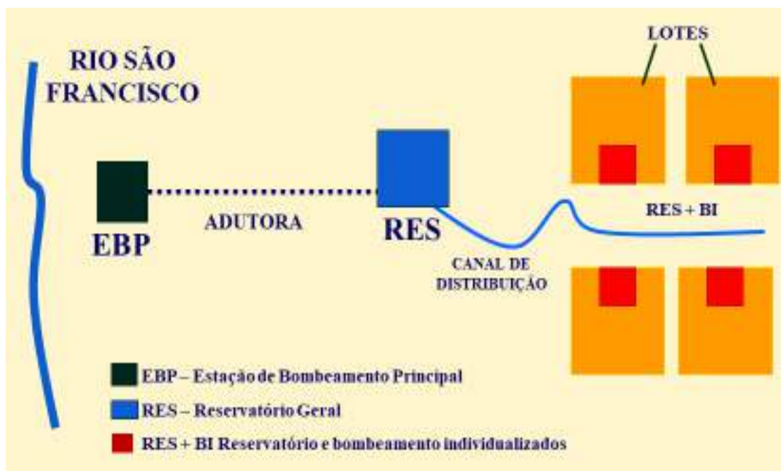
Figura 3. Modelo esquemático de funcionamento do projeto público de irrigação (PPI) Mandacaru após a conversão dos sistemas.
