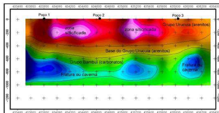
Figura 1. Perfil de eletro-resistividade do aquífero Urucuia sob em Luís Eduardo Magalhães (BA).
