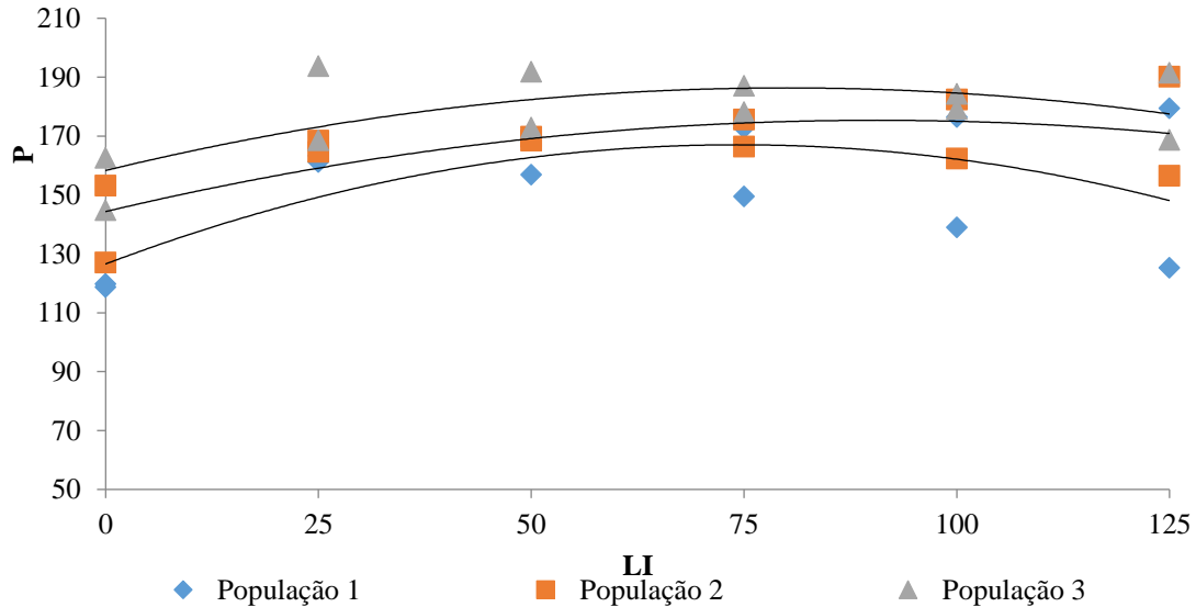
Figura 6. Produtividade do milho (P, sc ha -1 ) safrinha em função da lâmina de irrigação (LI, % ETc).
