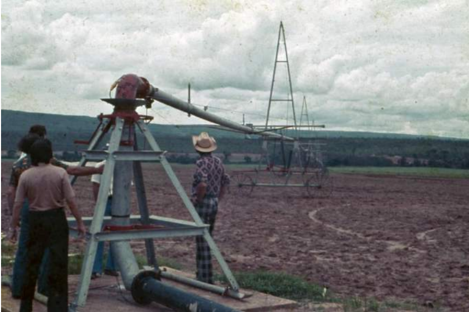
Figura 6. Primeiro pivô central importado, marca Valley, origem USA, instalado no Brasil, na Fazenda Chapadinha, município de Brasilândia/ MG, 1976 (foto disponibilizada por Fernando Antonio Rodriguez, 2020).
